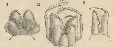
Fig. 5. Organos. - 1. Epeira. - 2. Tegenaria. - 3. Chivión
